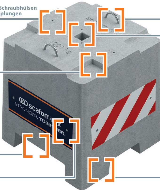
Aussparungen für verschiebesicheres Stapeln
