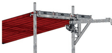
Рис. 39: V-образный кронштейн, конфигурация с внутренними консолями
