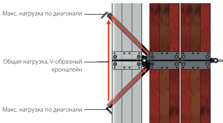
Рис. 40: Усилия, воздействующие на V-образный кронштейн
