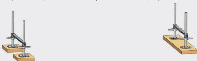
Рис. 3: Винтовые опоры с опорными поперечинами или поперечинами настила
