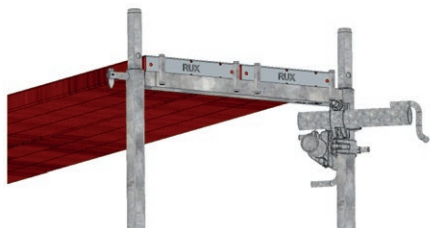
Рис. 38: V-образный кронштейн, базовая конфигурация
