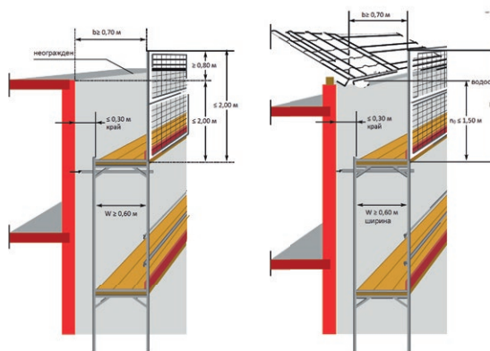
Рис. 59: Защитная стена с указанием размеров
