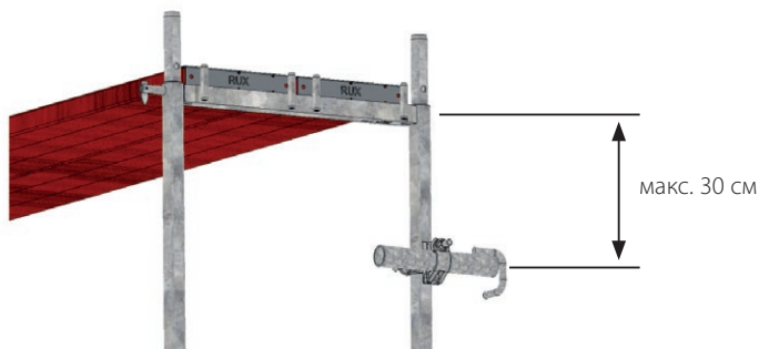
Рис. 43: Анкерные крепления с отличающимся положением анкеровки
