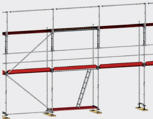
Рис. 29: Монтаж остальных единиц МЗП
