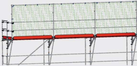
Рис. 61: Защитная стена на расширяющих консолях
