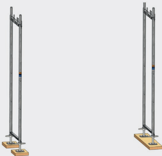
Рис. 6: Монтаж первой секции лесов: вертикальные рамы
