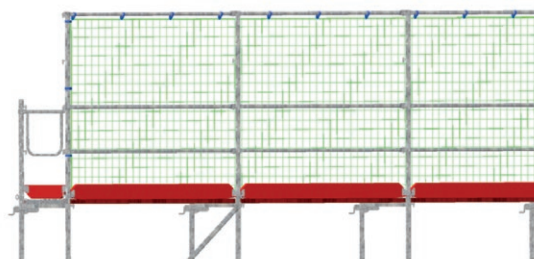
Рис. 60: Защитная стена на вертикальных рамах
