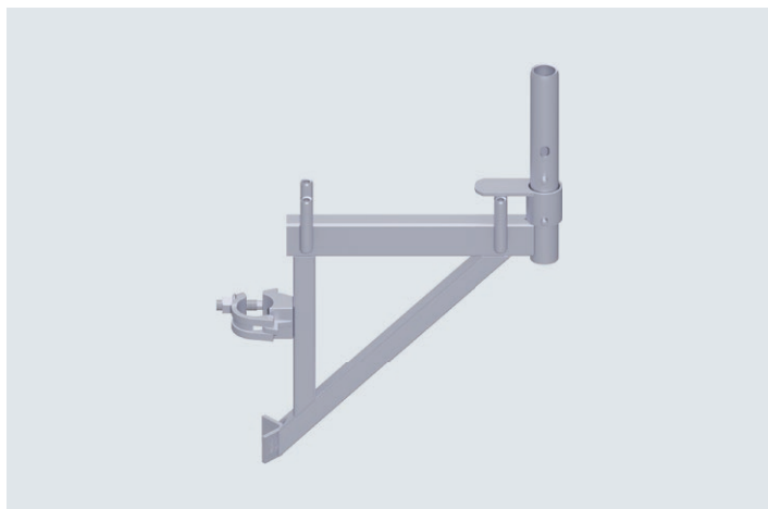
Konsole PLEX 32
