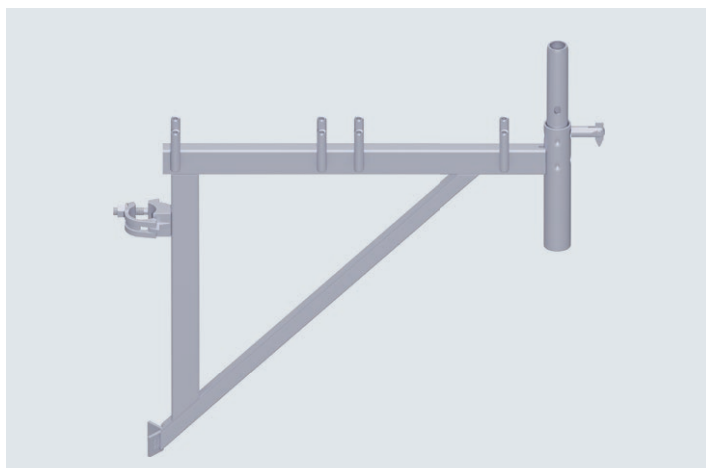
Konsole PLEX 64
