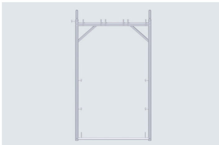
Stahl-Vertikalrahmen PLEX 110 H 200 cm, 4 Kippstifte
