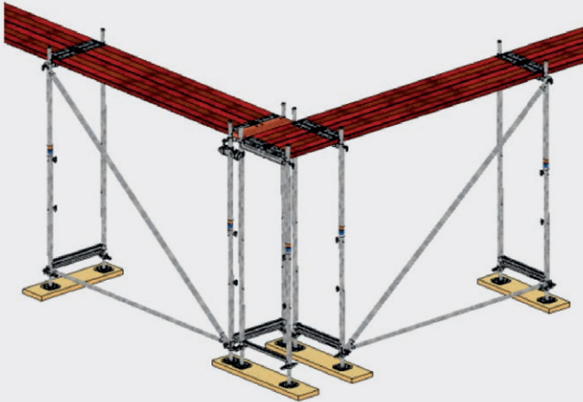
Bild 19: ECKAUSBILDUNG mit drei Vertikalrahmen
