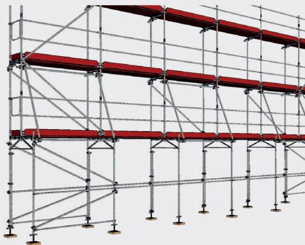
Bild 53: Durchgangsrahmen
