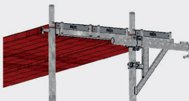
Bild 37: Kurzer Gerüsthalter, Ausführung mit Verbreiterungskonsolen innen
