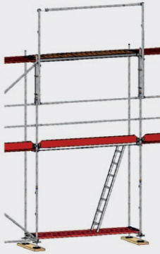
Bild 28: Einhängen des zweiten MSG-Pfosten.
