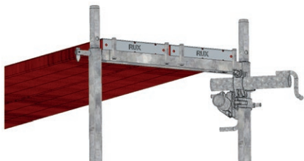
Bild 38: V-Halter, Grundkonfiguration
