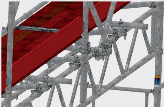
Bild 57: Anschluss der Diagonalen mit Normalkupplungen
