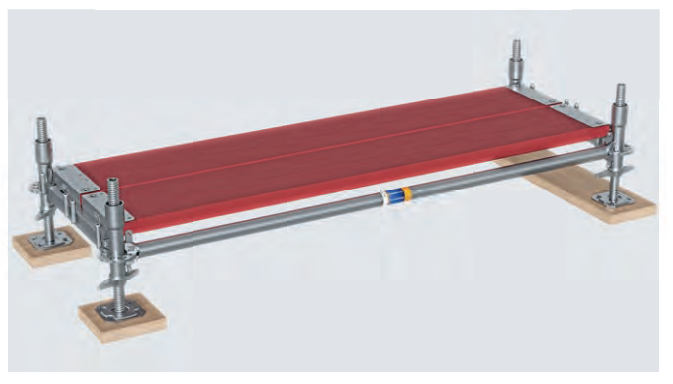
Bild 22 Belagbohlen auf Belagriegel
