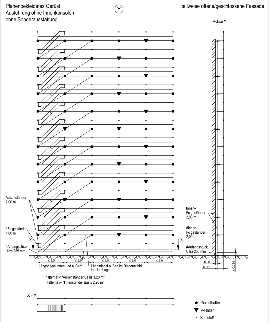
Bild 92 Planenbekleidetes Gerüst: Ausführung ohne Innenkonsolen ohne Sonderausstattung, teilweise offene/geschlossene Fassade
