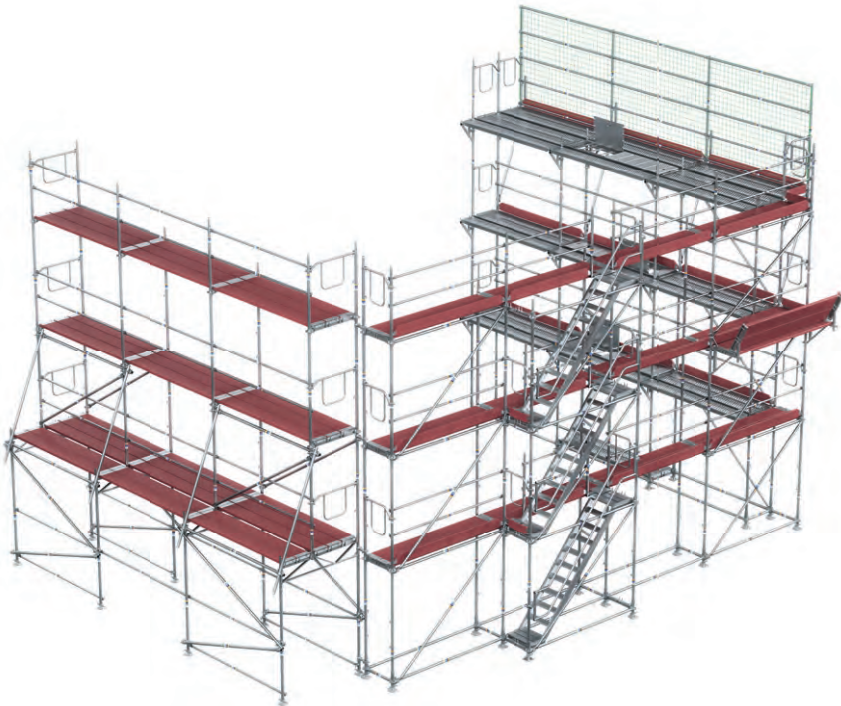
Bild 9 Übersicht SUPER-RS
