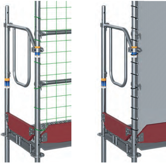
Bild 66 Bekleidung mit Netzen und mit Planen
