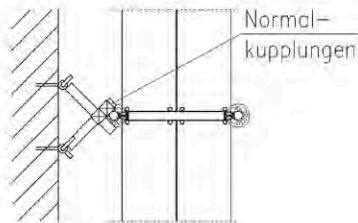
Bild 79 Verankerung: Details
