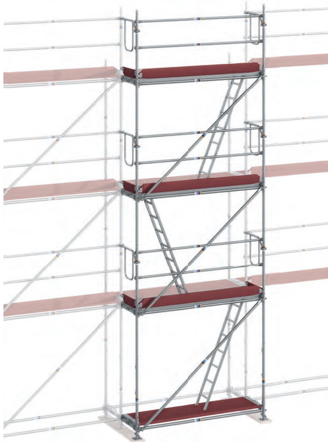
Bild 48 Vorgestellter Leiteraufstieg
