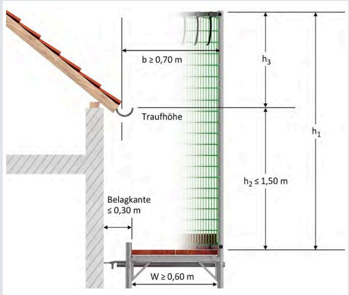
Bild 6 Schutzwände (geneigte Dächer)
