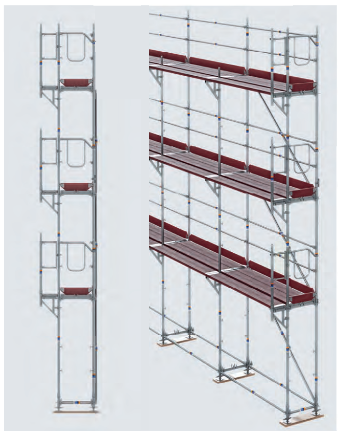
Bild 50 Gerüst mit Verbreiterungskonsolen innen
