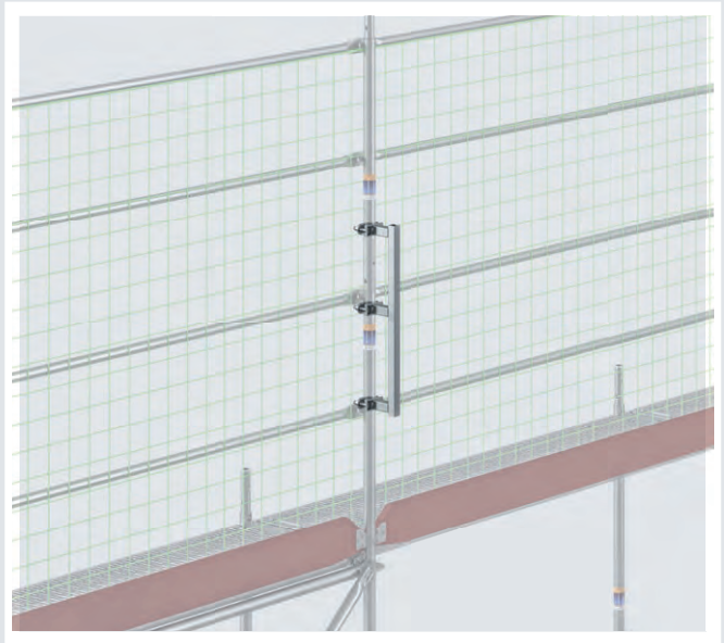
Bild 62 Geländerständer-Sicherung für Schutznetze (gerade)
