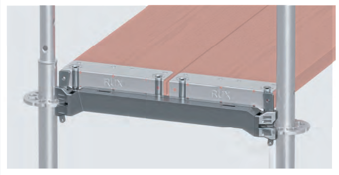
Bild 11 Belagriegel mit Zapfen
