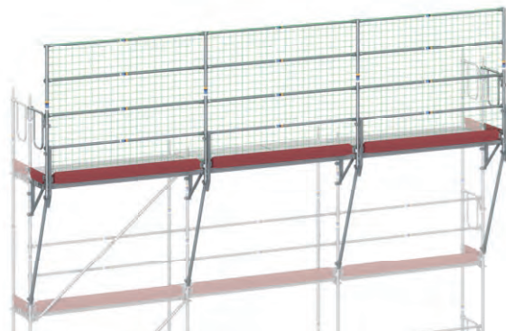
Bild 65 Schutzwand auf Verbreiterungskonsolen
