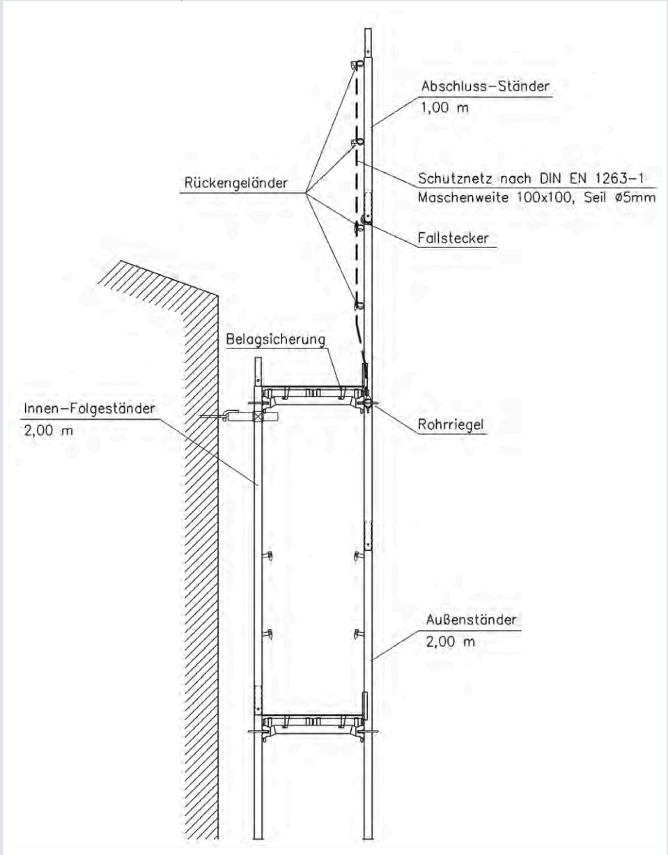
Bild 78 Schutzwand: Details
