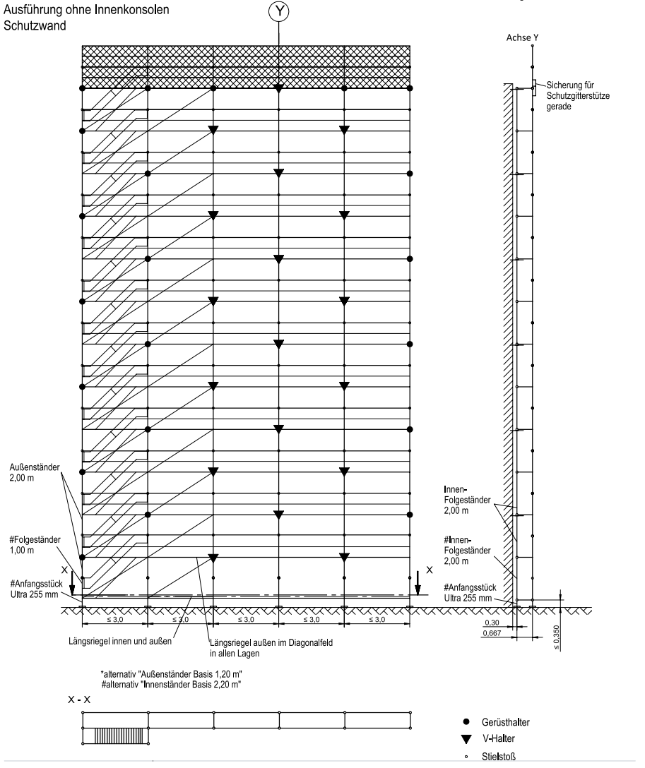
Bild 85 Netzbekleidetes Gerüst: Ausführung ohne Innenkonsolen, Schutzwand, geschlossene Fassade
