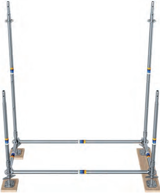
Bild 25 Aufbau mit Innenständer 2,00 m und Außenständer 1,00 m mit Kippstift mit RINGSCAFF-Anfangsstück
