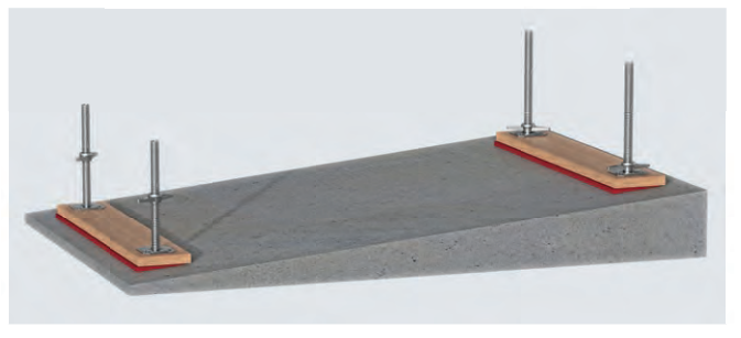
Bild 18 Unterbau auf geneigtem Untergrund
