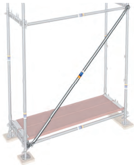
Bild 29 Einbau Vertikaldiagonale
