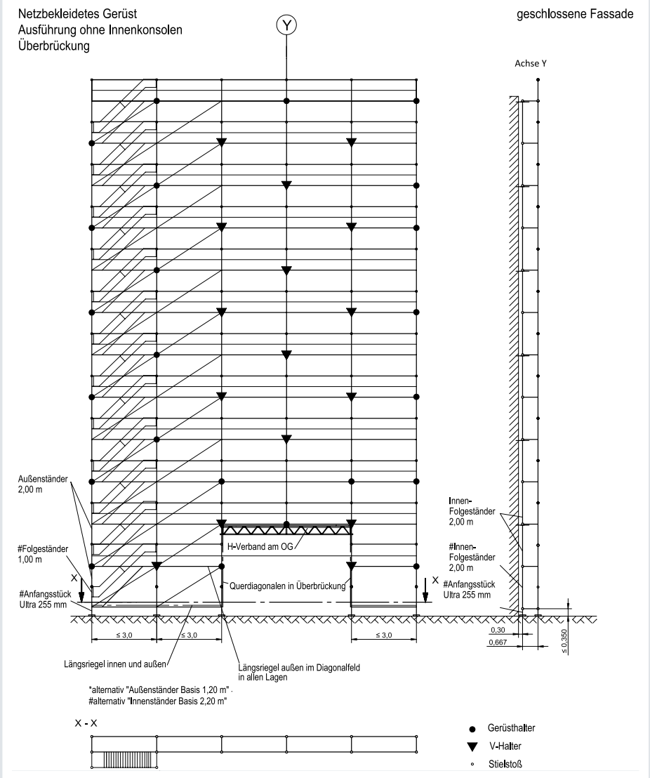
Bild 89 Netzbekleidetes Gerüst: Ausführung ohne Innenkonsolen, Überbrückung, geschlossene Fassade
