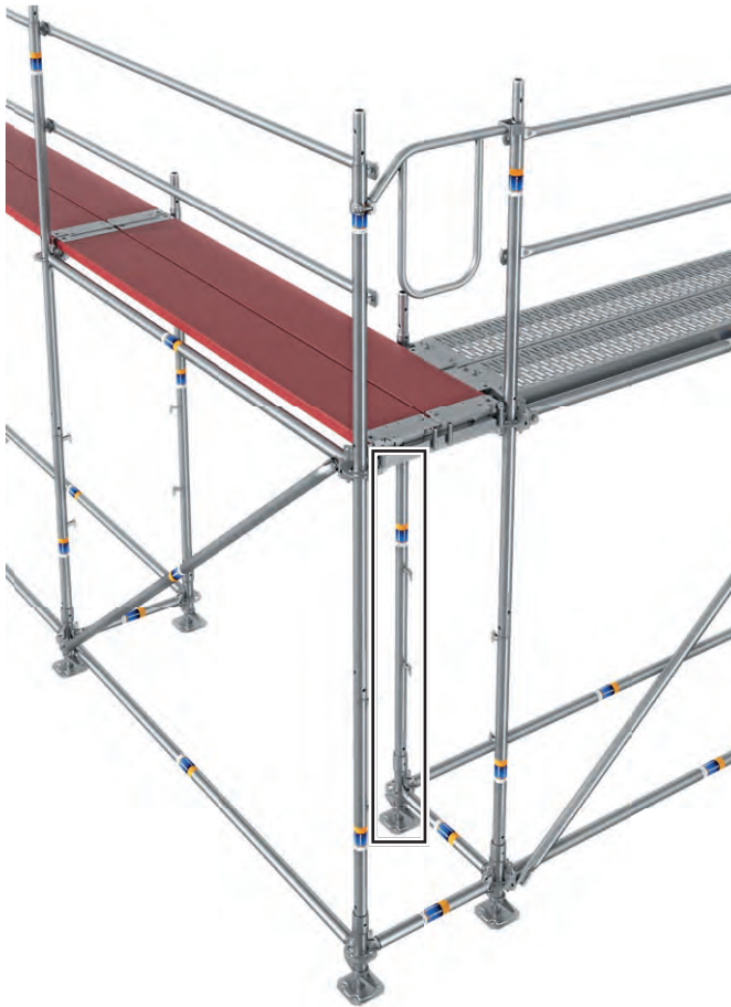
Bild 38 ECKbildung von 2 Gerüstsebenen um 90° (Eckständer)
