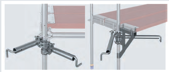
Bild 41 V-Halter Grundkonfiguration und Konfiguration mit Innenkonsolen
