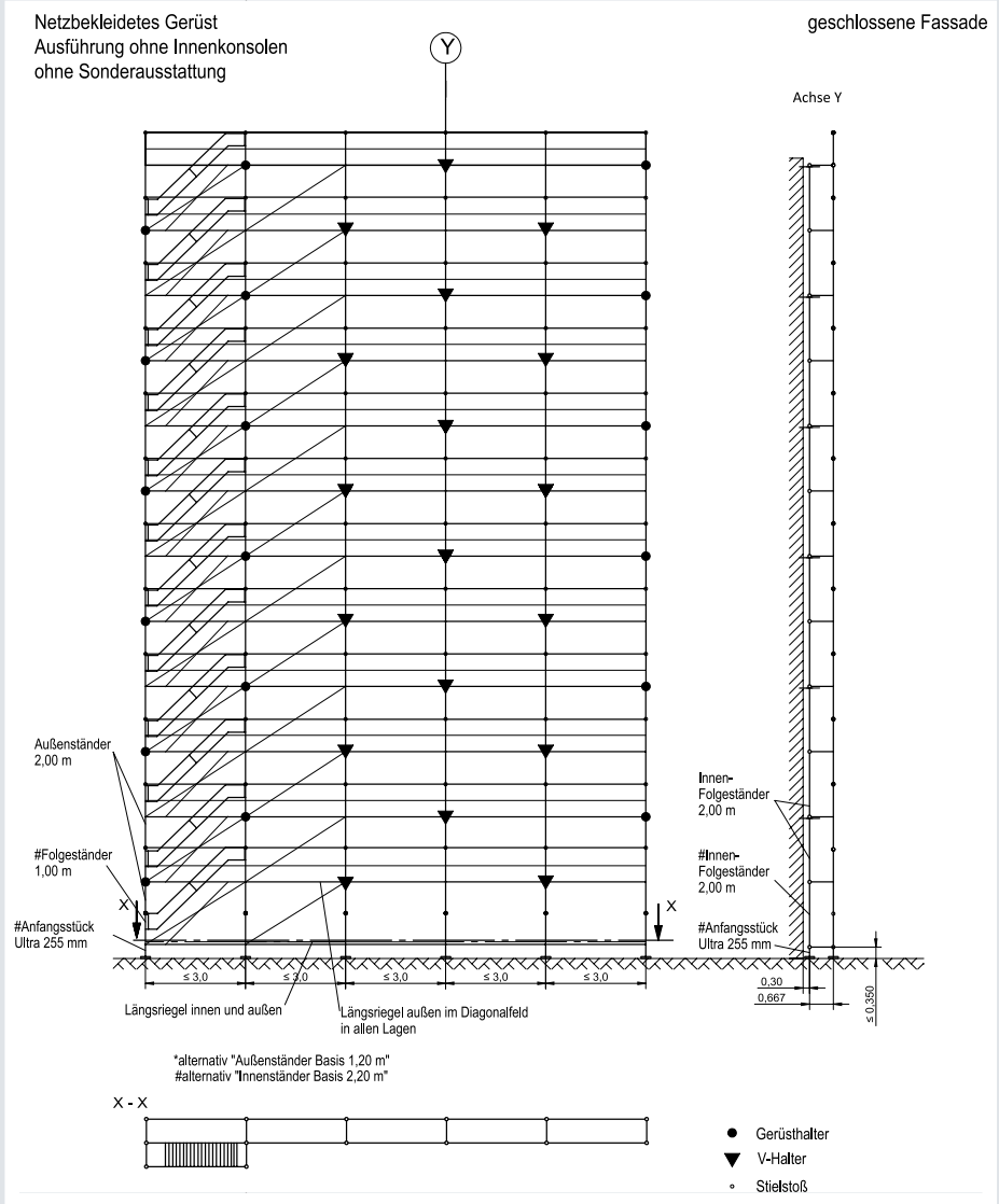
Bild 81 Netzbekleidetes Gerüst: Ausführung ohne Innenkonsolen, ohne Sonderausstattung, geschlossene Fassade
