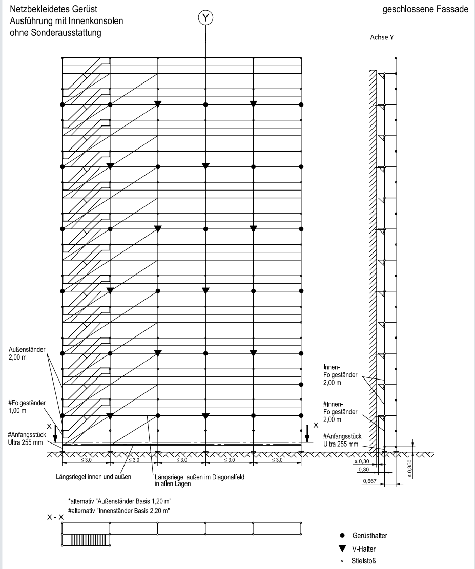
Bild 83 Netzbekleidetes Gerüst: Ausführung mit Innenkonsolen, ohne Sonderausstattung, geschlossene Fassade
