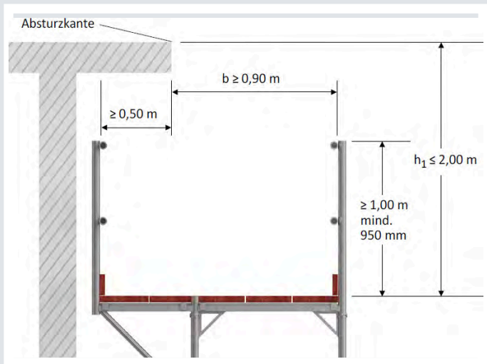
Bild 4 Fanggerüst bei überstehender Absturzkannte und Belagbreite über 0,90 m
