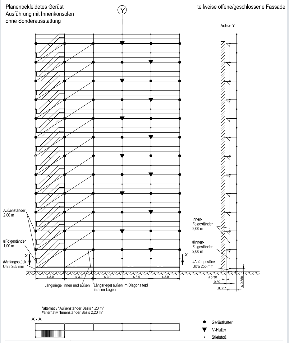
Bild 94 Planenbekleidetes Gerüst: Ausführung mit Innenkonsolen, ohne Sonderausstattung, teilweise offene/geschlossene Fassade
