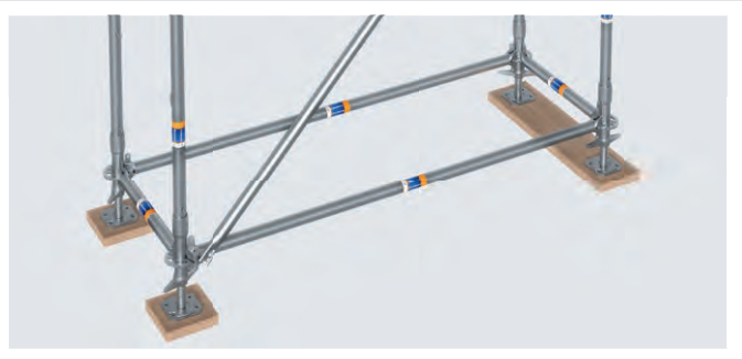
Bild 23 Längsriegel
