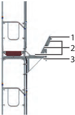
Bild 61 Schutzdach
