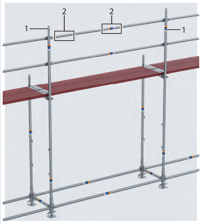
Bild 2 Zulässige Anschlagpunkte für die PSAGa
