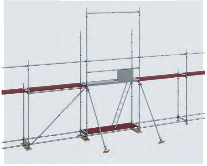
Bild 7 Vorübergehende Kippsicherung der ersten Gerüstebene
