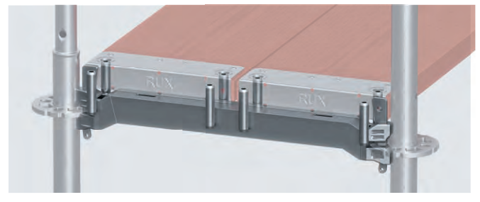
Bild 33 Belagriegel
